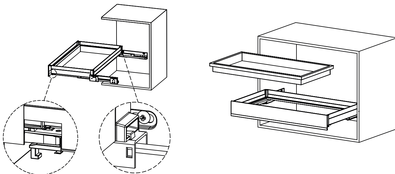
Схема системы, установленной в корпус
