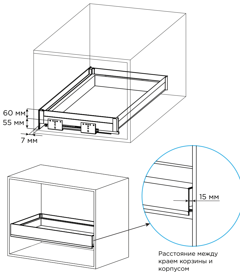
Схема системы, установленной в корпус
